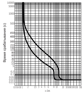
Рисунок 2б - Времятоковые характеристики выключателей BA88-32M с ln>32A
