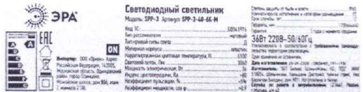
Маркировка светильника
