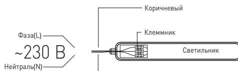
Рис. 1. 230В шамчыракты токко туташтыруу схемасы
