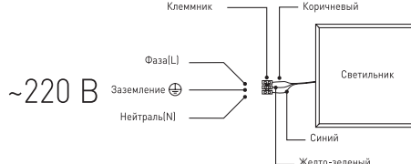
Рис.1. 220В шамчыракты токто туташтыруу схемасы
