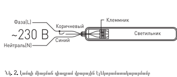
Նկ. 2. Լամպի միացման դիագրամ վրաբային էլեկտրամատակարարմամբ
