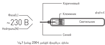
Նկ.1 կամպը 230Վ, ցանցին միացնելու սխեմա
