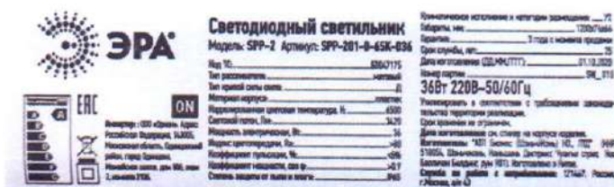
Маркировка светильника
