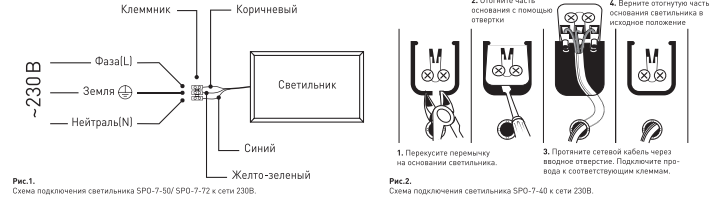
Рис.1. Схема подключения светильника SPO-7-50/ SPO-7-72 к сети 230В.
