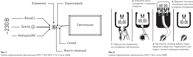
Рис.1. Схема подключения светильника SPO-7-50/ SPO-7-72 к сети 230В.
