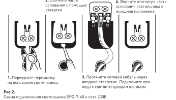
Рис.2. Схема подключения светильника SPO-7-40 к сети 230В.
